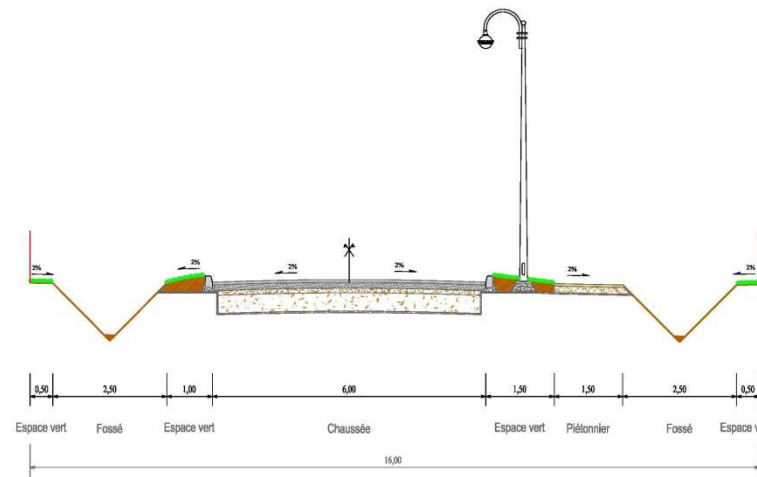
Coupe type de la voirie
